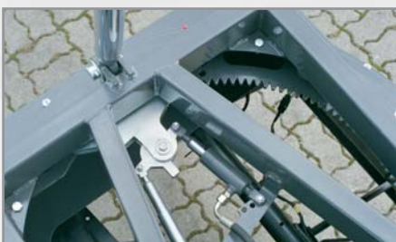
Stufenlose, hydraulisch lösbare Drehkranzsperr
