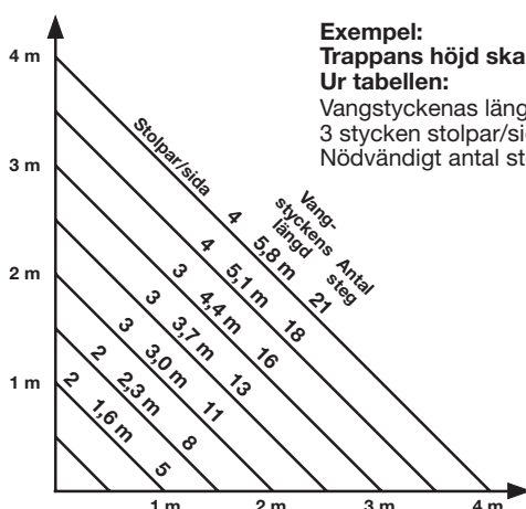
Beräkning av vangstycken, antal steg och stolpar
